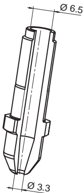
Tip seat - Siege de pointe - Einbaumaße
