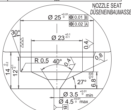
PIN SHUT OFF SEAT CONICAL KONISCHE NADELABDICHTUNG
