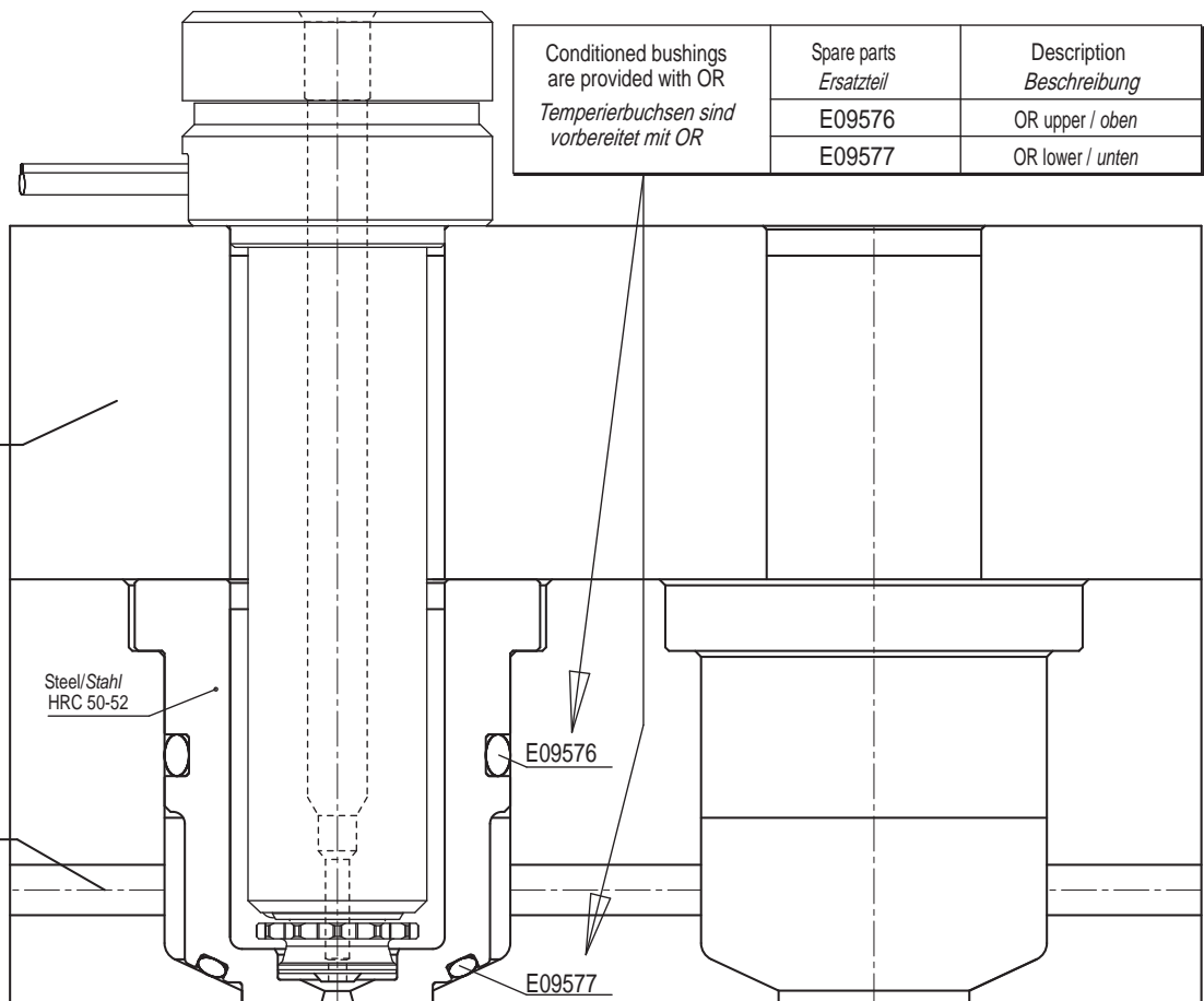
BUSHING + NOZZLE / VORKAMMER + DÜSE BUSHING SEAT / EINBAUMAßE FÜR VORKAMMERBUCHSE
