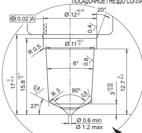
NOZZLE SEAT ПОСАДОЧНОЕ ГНЕЗДО СОПЛА
