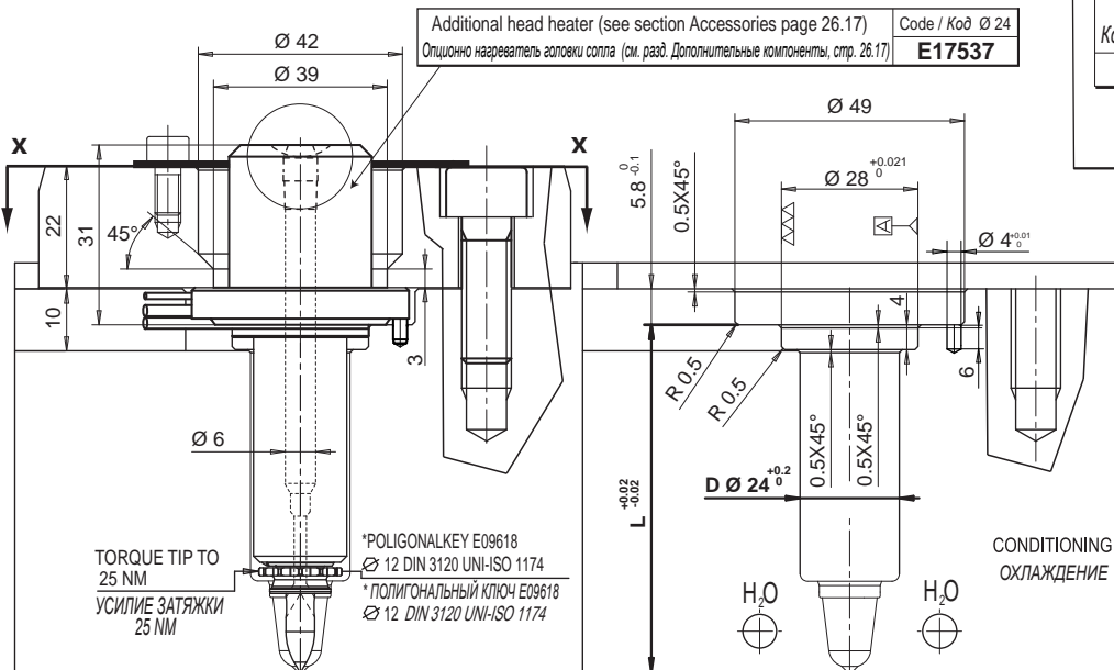
NOZZLE СОПЛО
